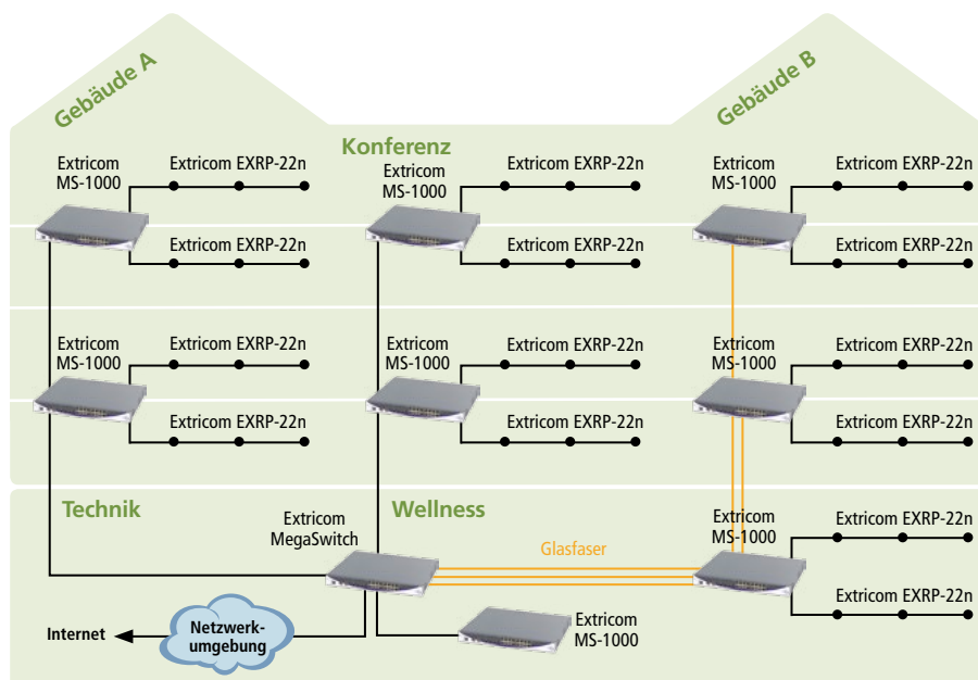
Beispielszenario Hotel mit Extricom WLAN: Bis zu 8 MS-1000 Switches werden an den MegaSwitch angeschlossen.
